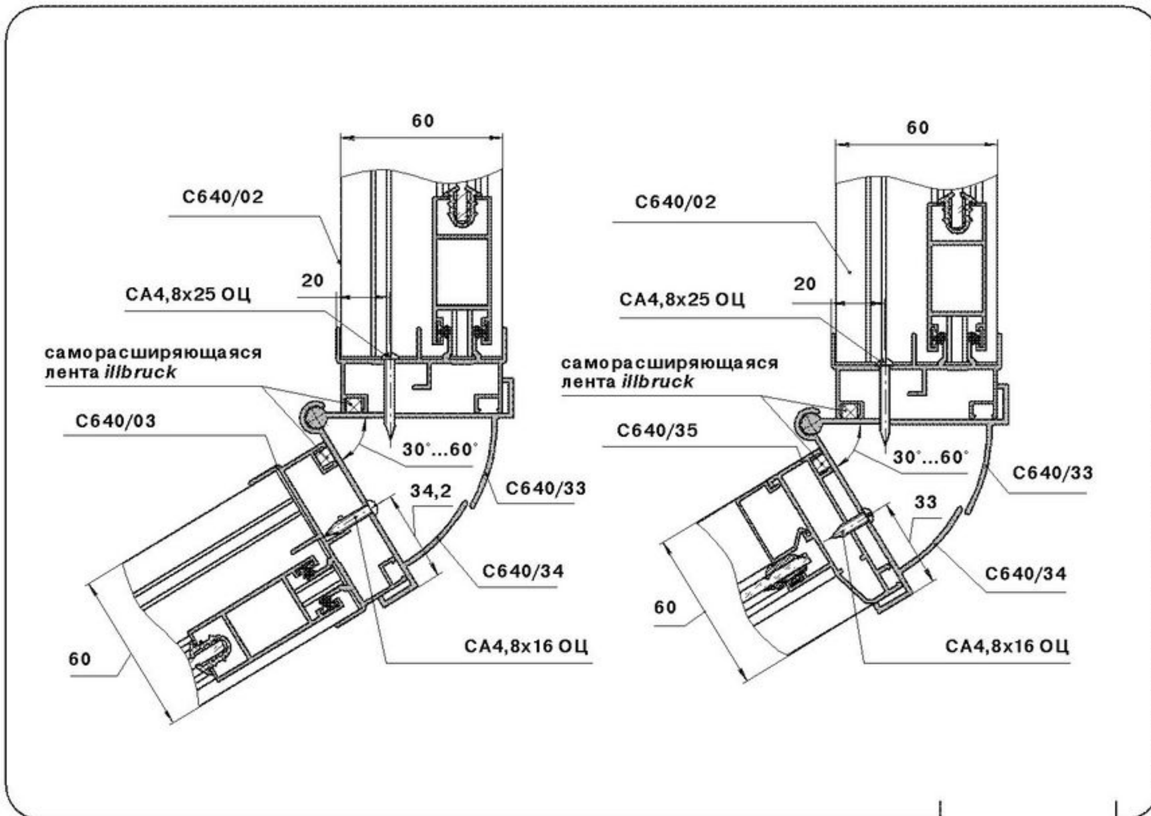
узел 1
